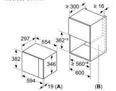
A: 20 mm para frente metálica B: Parede traseira aberta
